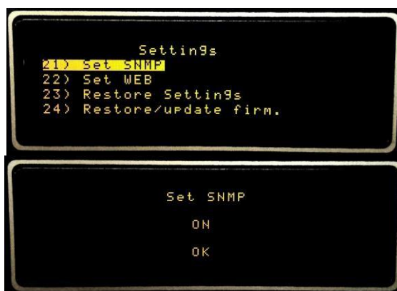
Рисунок 21 — Настройка SNMP
