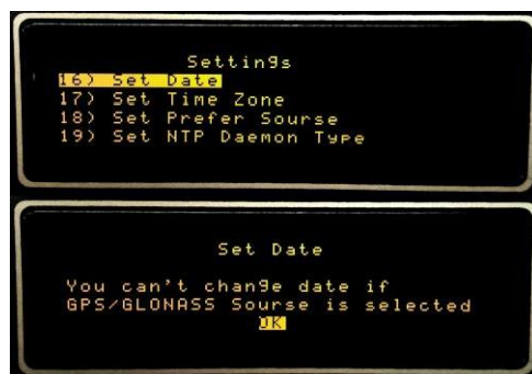
Рисунок 16 — Настройка Даты
