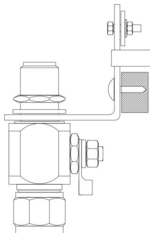
Рисунок 3.4 Крепление грозоразрядника
