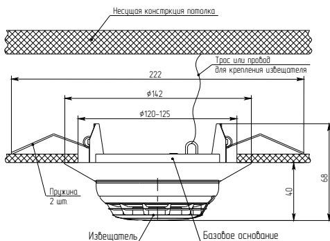
Рисунок 2 – Установка извещателя на подвесном потолке
