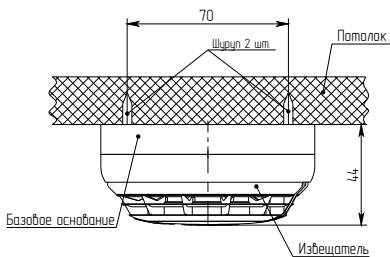
Рисунок 1 – Установка извещателя на потолке
