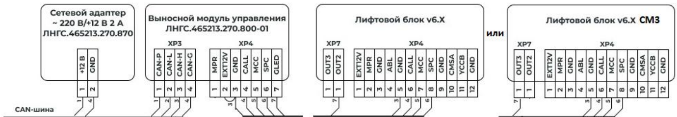
Рисунок Б.2 – Подключение ВМУ к ЛБ6.X
