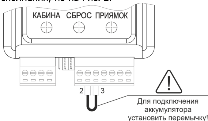
Рисунок 2 – Подключение аккумуляторной батареи ВМУ
