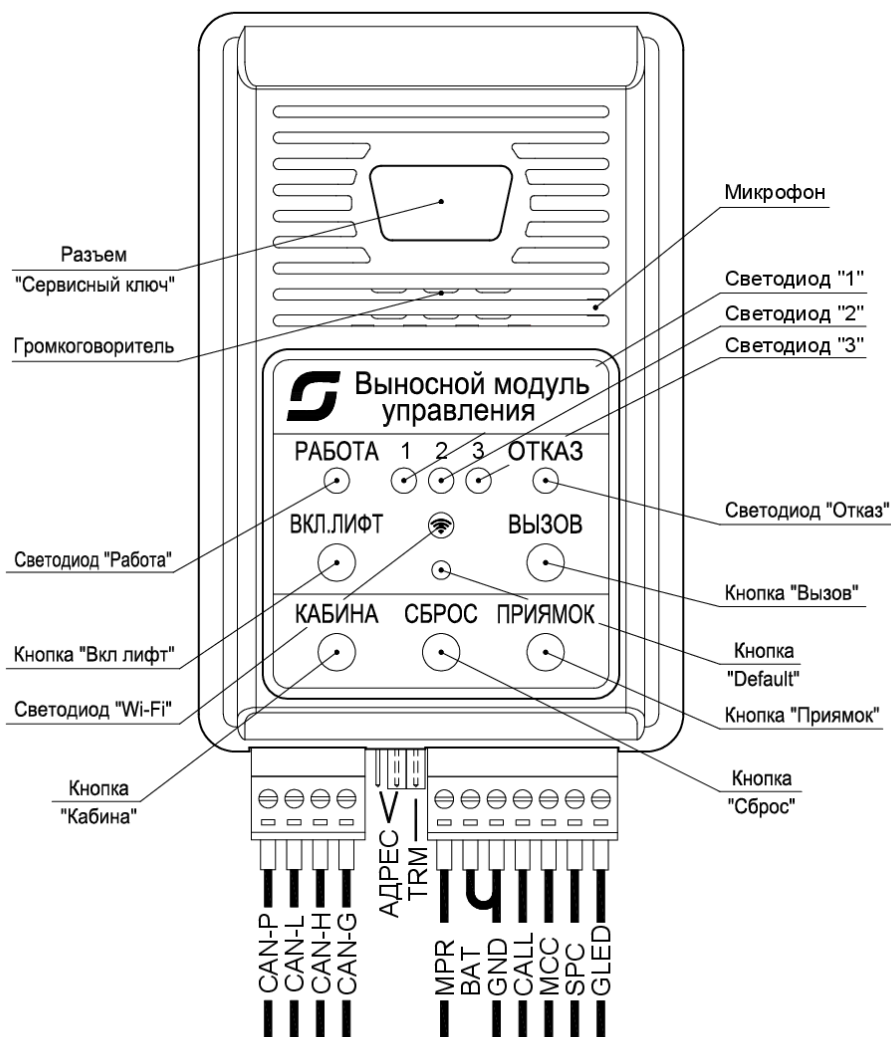
Рисунок 1 – Внешний вид ВМУ, назначение разъемов, органов управления и индикации
