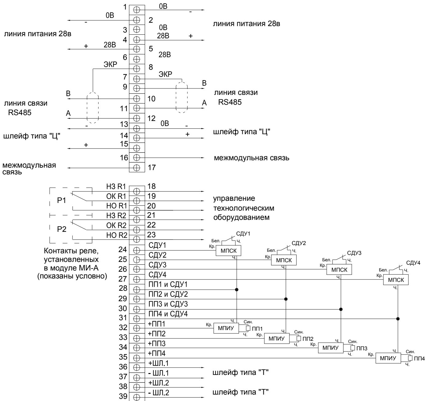
Рисунок 1 – Схема подключения модуля МИ-А исп. К
