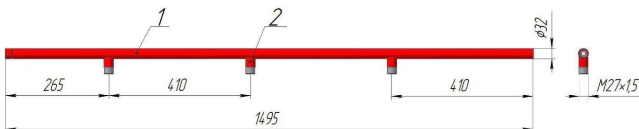
Рисунок 5.15 – Коллектор однорядный для подключения трёх модулей объёмов 60, 80 или 100 литров серий «АТАКА 1» и «АТАКА 2», а также модуля типа МГПи серии «АТАКА»
