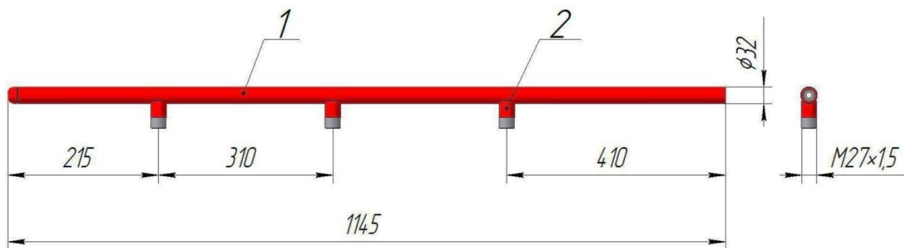
Рисунок 5.14 – Коллектор однорядный для подключения трёх модулей объёмом 40 литров всех серий
