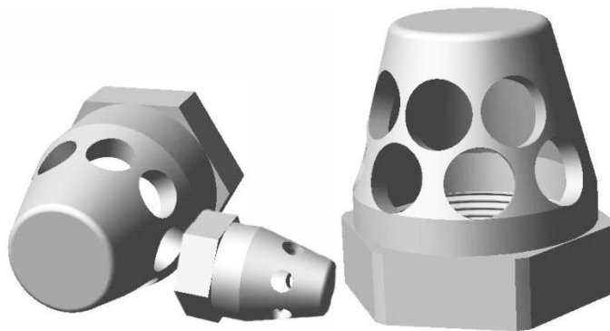
Рисунок 5.3 – Общий вид газовых распылителей
