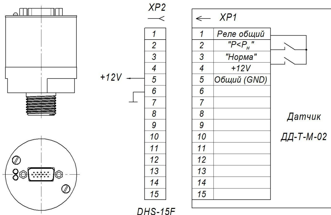
Рисунок 8.2 – Электрическая схема подключения датчика давления DD-T-M-02
