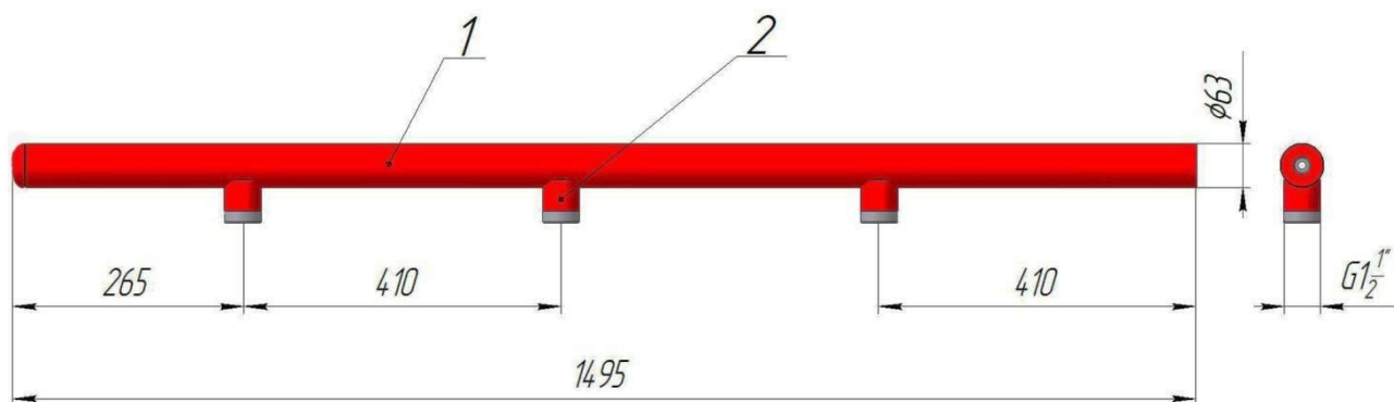
Рисунок 5.13 – Коллектор однорядный для подключения трёх МГП 60 и МГП 65 объёмов 60, 80 или 100 литров серии «АТАКА»
