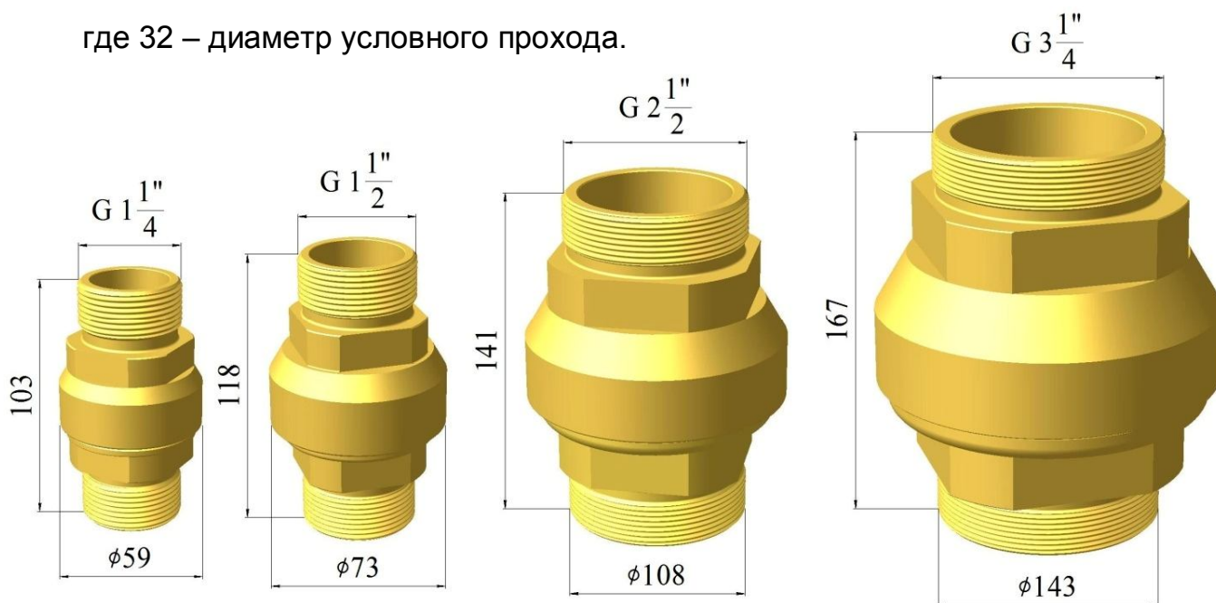
Рисунок 7.1 – Обратные клапаны КО-25, КО-32, КО-50 и КО-70
