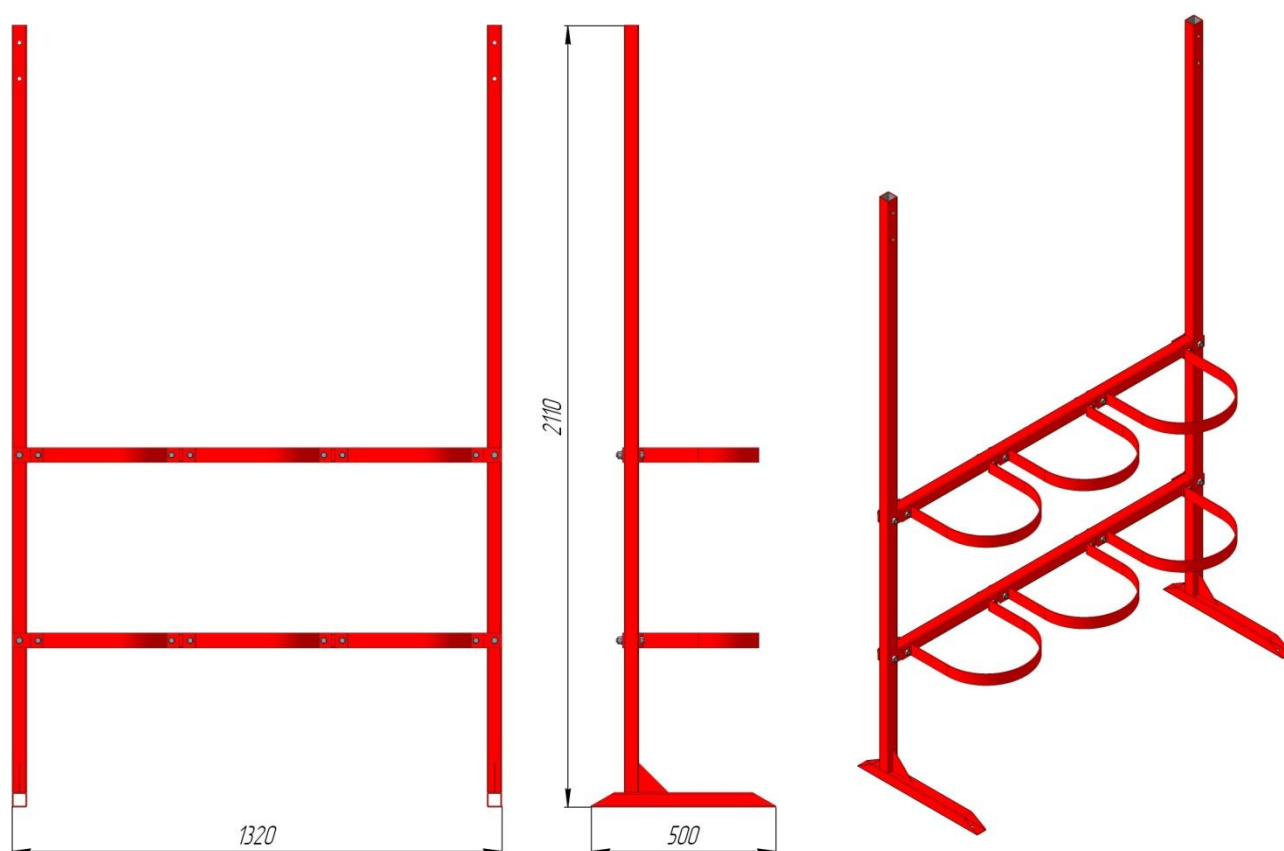
Рисунок 4.12 – Рама для трёх модулей типа МГП (60-80-32) «АТАКА»
