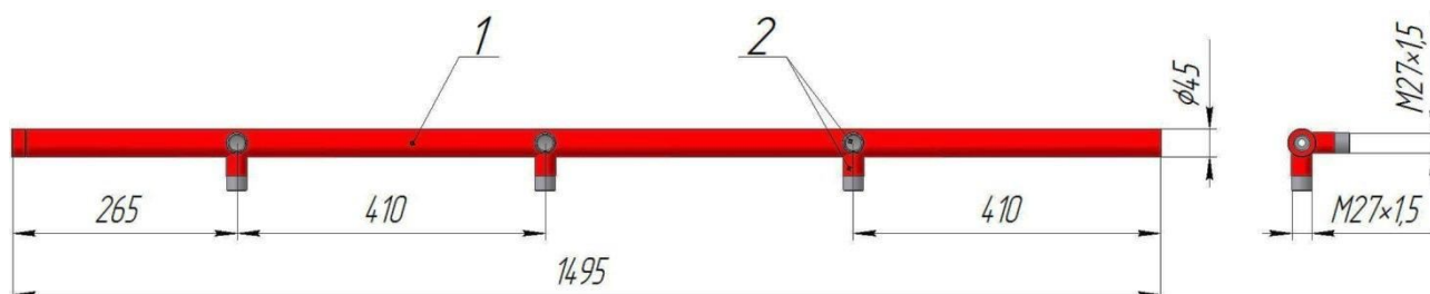
Рисунок 5.16 – Коллектор двухрядный для подключения шести модулей объёмов 60, 80 или 100 литров серий «АТАКА 1» и «АТАКА 2», а также модулей типа МГПи серии «АТАКА»
