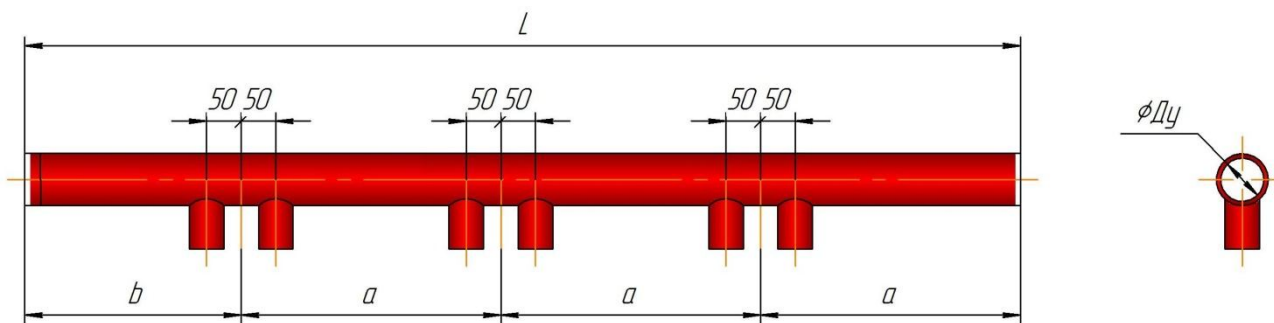
Рисунок 5.11 – Устройство коллектора для двухрядной батареи, основанной на МГП 60 и МГП 65
