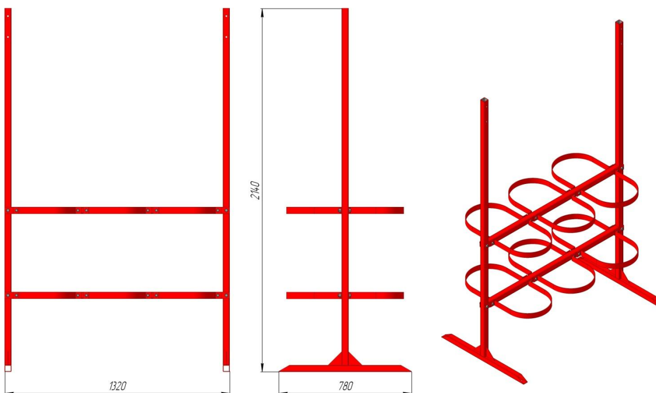
Рисунок 4.13 – Рама для шести модулей типа МГП (60-80-32) «АТАКА»
