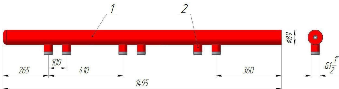
Рисунок 5.17 – Коллектор однорядный для подключения шести МГП 60 и МГП 65 объёмов 60, 80 или 100 литров серии «АТАКА»
