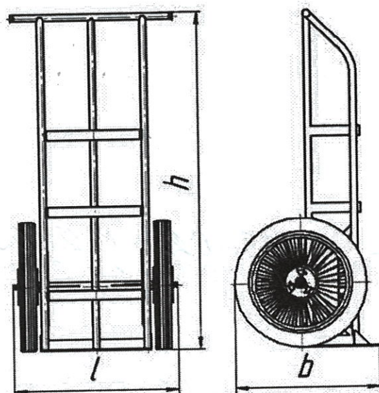
Рис. 23.9 Тележка транспортная
