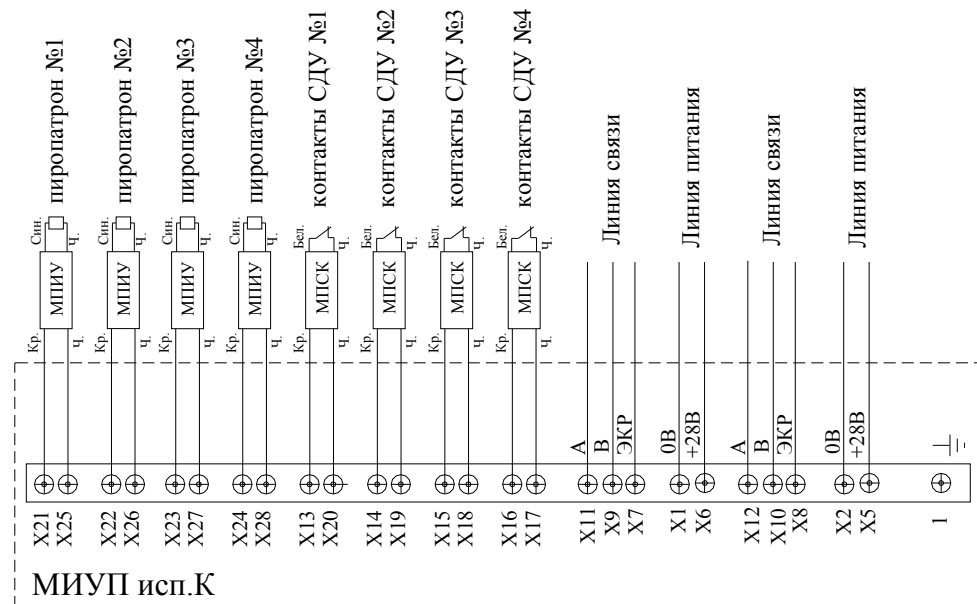
Рисунок 1 – Схема подключения модуля МИУП исп. К
